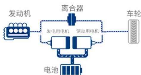
图 23：本田 i-MMD 混动系统构型原理图
