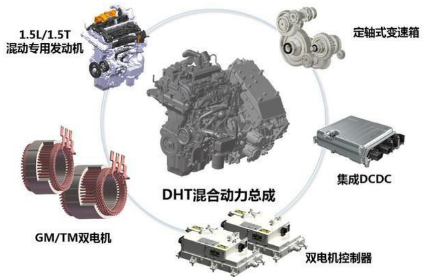
图 35：长城柠檬七合一 DHT 混合动力系统总成
