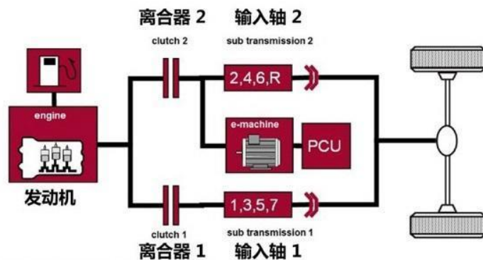
图 45：吉利 P2.5 构型混动系统 ePro
