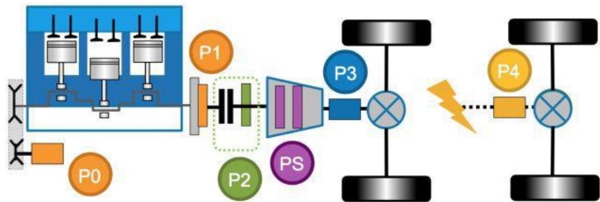
图 12：混合动力系统不同的电机位置
