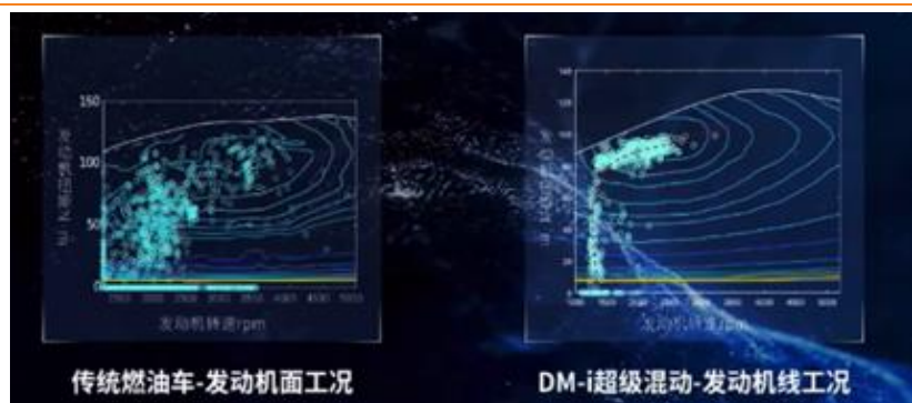
图 12 月：比亚迪 DM-i 混动系统的发动机工作点与传统燃油车对比
