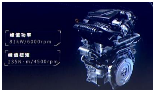
图 27：比亚迪 DM-i 搭载的骁云插混专用发动机
