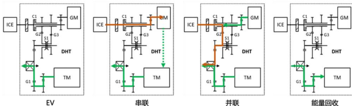
图 38：长城柠檬 DHT 混动系统的工作模式
