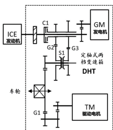
图 36：长城柠檬 DHT 混动构型
