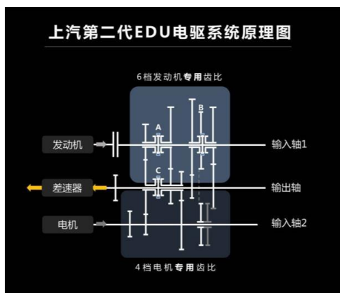
图 42：上汽 EDU Gen2 混动系统构型
