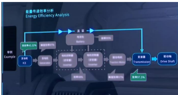
图 51：DHT Pro 能量传递图
