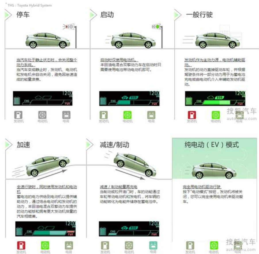
图 20：THS 系统行驶时工作模式
