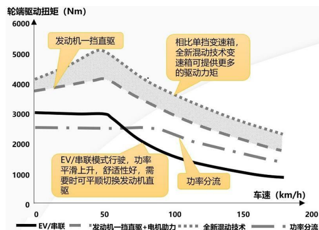
图 37：长城柠檬 DHT 混动的模式切换逻辑
