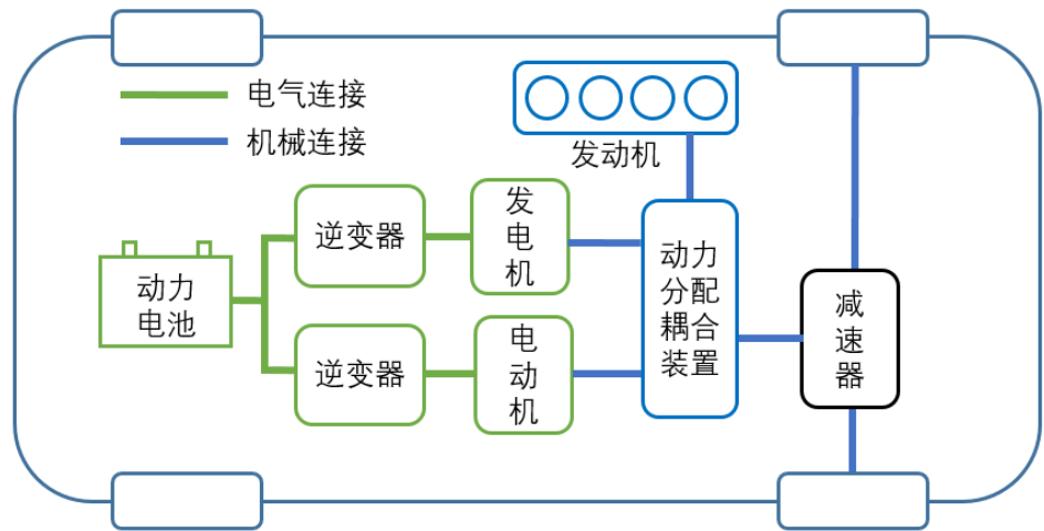
图 15：混联（串并联）构型原理图
