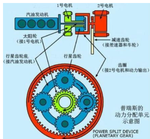
图 19：丰田 THS 混动系统构型原理
