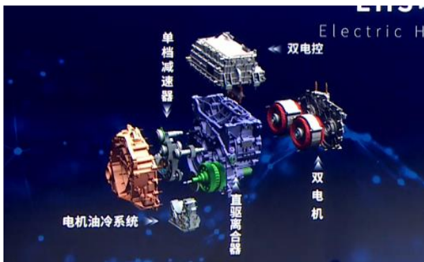
图 26：比亚迪 DM-i EHS 电混构型
