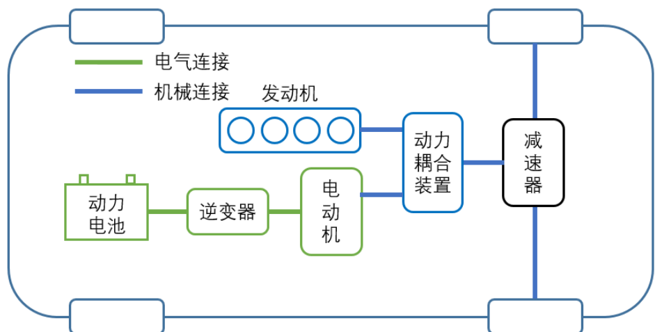
图 14：并联构型原理图
