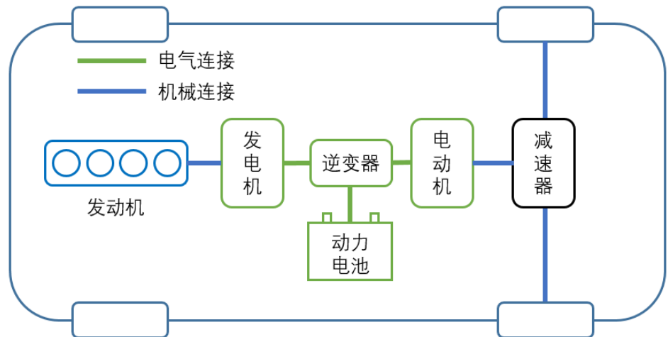
图 13：串联构型原理图
