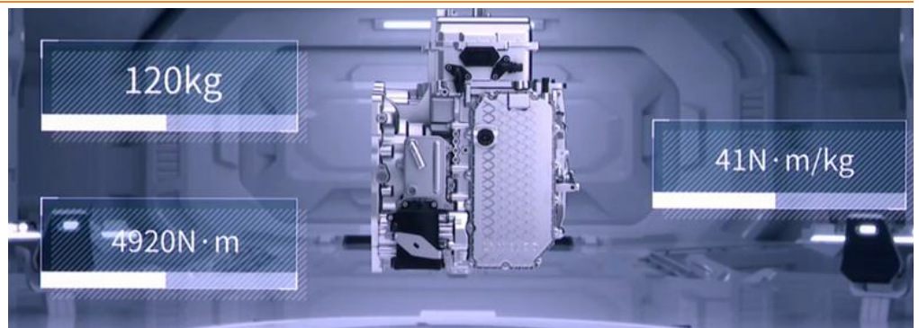
图 53：DHT Pro 混动专用变速箱参数
