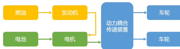
图 7：混动汽车工作模式—串联驱动
