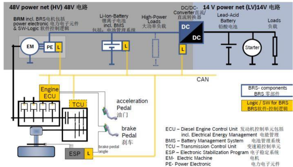
图 16: Bosch 48V 混动系统技术方案
