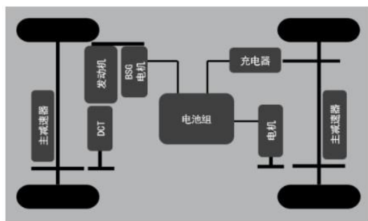
图 31：比亚迪 DM-p 双擎四驱原理
