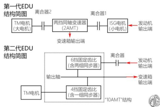
图 43：上汽两代混动系统差异对比
